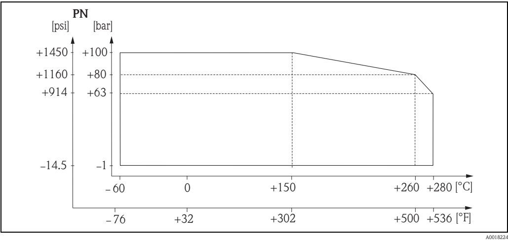
高压型滑动套管的压力 - 温度曲线
